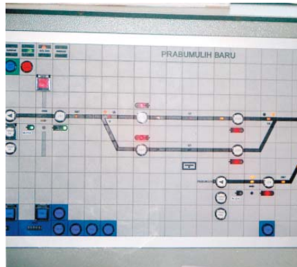
ALAT MONITOR: Perjalanan kereta api di Prabumulih Baru, Sumatera Selatan.
