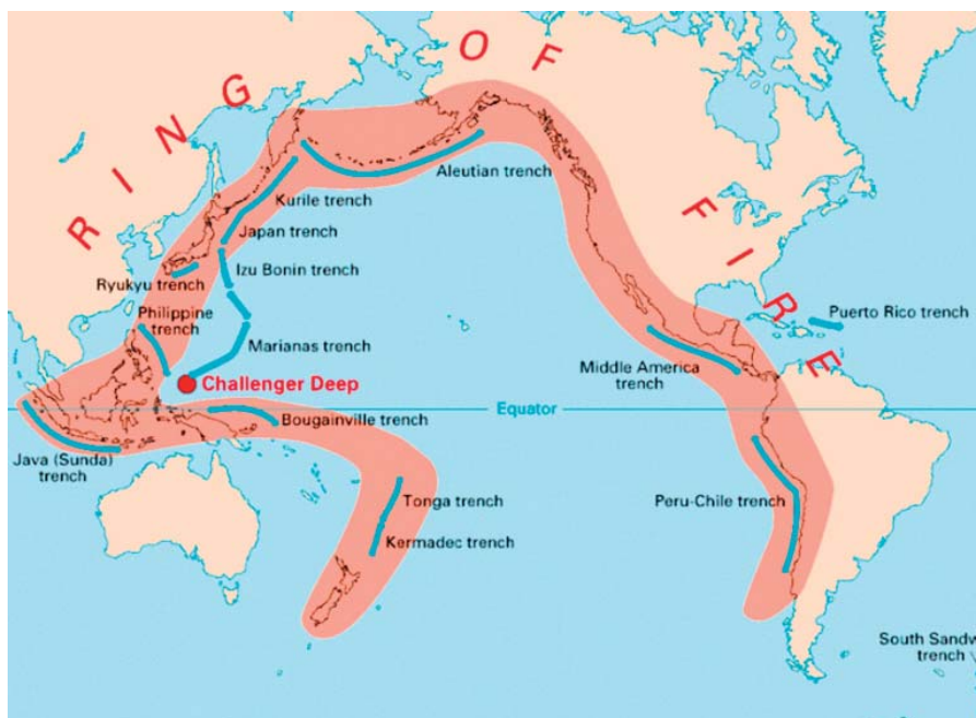
RING OF FIRE: Empat lempeng aktif bersinggungan dengan Indonesia.
